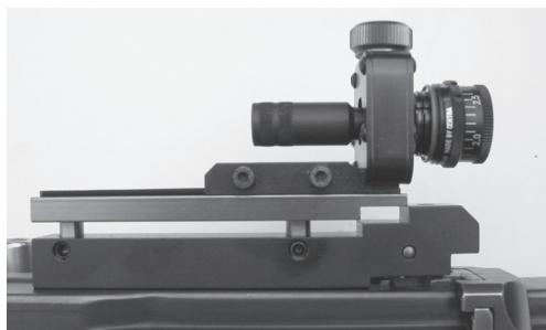
Figura 13: Supporto dell'alzo per il F ass 57 per il montaggio di comuni alzi circolari resistente agli urti e/o contraccolpi – rinculo diversi modelli
